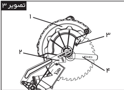
۱. صفحه ثابت محافظ ایمنی ۲. محافظ متحرک ۳. پیچ ۴. آچار
