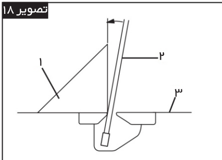
۱. گونیا ۲. تیغه اره ۳. میز پایه چرخش
