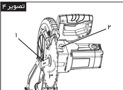
۱. پیچ ۲. کلید قفل کن ۳. باز کردن
